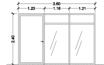
ELEVÇÃO 02 ESC: 1:75
