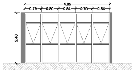
ELEVAÇÃO 01 ESC: 1:75
