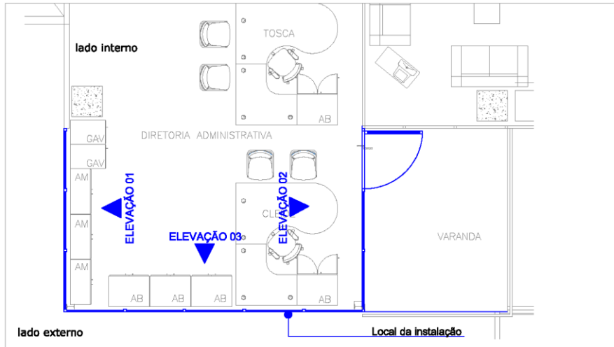
PLANTA DE LOCALIZAÇÃO - SALA DIRETORIA ADMINISTRATIVA - 4º PAV. ESC: 1:75
