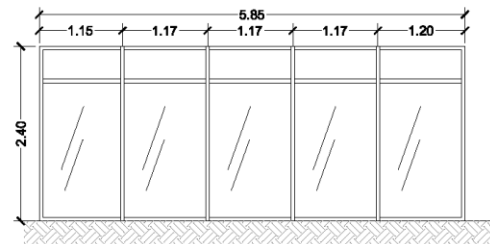
ELEVÇÃO 03 ESC: 1:75
