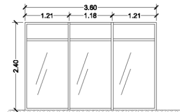
ELEVÇÃO 01 ESC: 1:75
