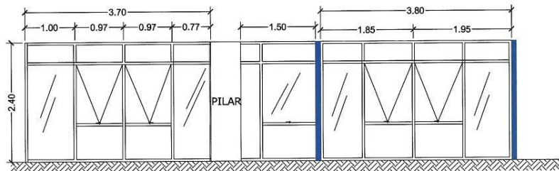
ELEVÇÃO 01 ESC: 1:75
