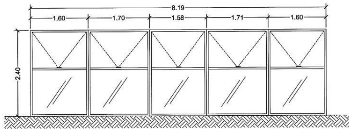
ELEVAÇÃO 02 ESC: 1:75
